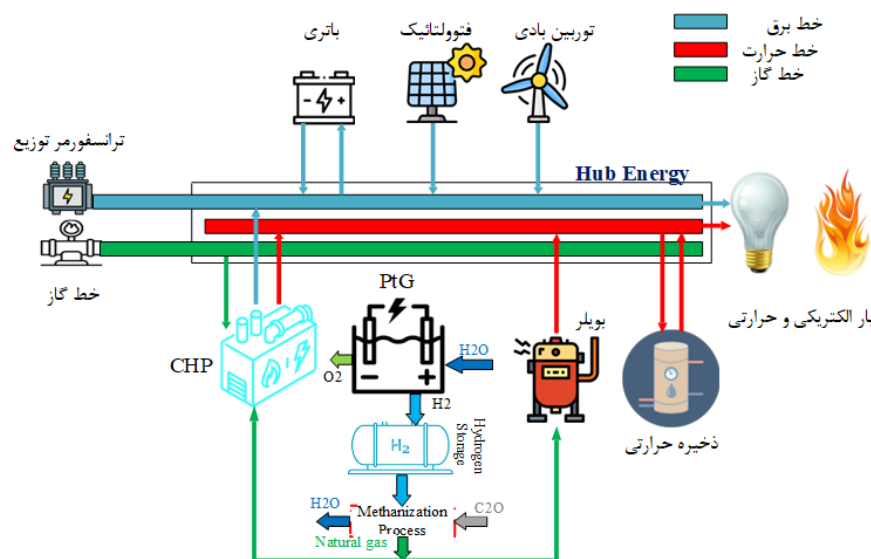
شکل (۱): توپولوژی پیشنهادی هاب انرژی Figure (1): Proposed Energy Hub Topology
