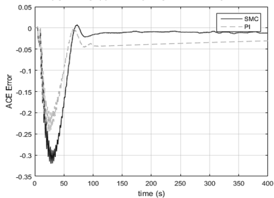
شکل (۹): خطای کنترل ناحیه (ACE) در ناحیه دوم برای سناریو ۱
