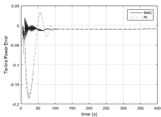
شکل (۷): خطای توان خط ارتباطی در ناحیه اول برای سناریو ۱
