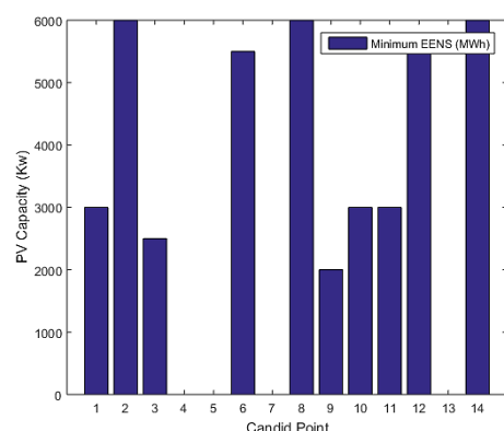
شکل (۵): ظرفیت نصب شده در نقاط کاندید در عضوی با کمترین میزان EENS
