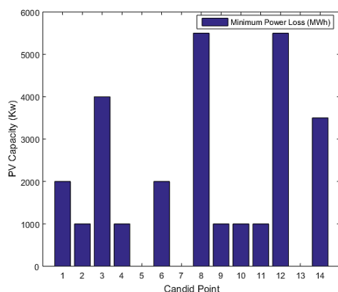
شکل (۴): ظرفیت نصب شده در نقاط کاندید در عضوی با کمترین تلفات انرژی
