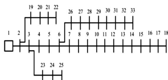
شکل (۲) شبکه ۳۳ شینه تحت استاندارد IEEE
