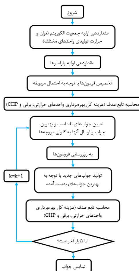
شکل (۱): فلوچارت الگوریتم روش پیشنهادی
