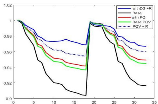
شکل (۶) پروفیل ولتاژ در شبکه ۳۳ شینه در حالت‌های مختلف
