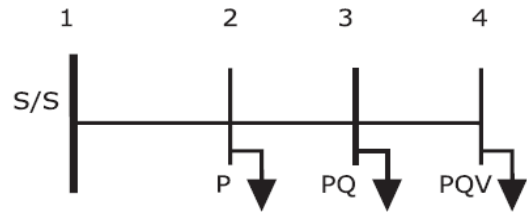
شکل ۱ یک نمونه چهار شینه شبکه توزیع نشان دهنده شین های P و PQV است.
