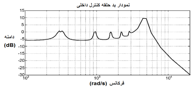
شکل (۱۰): نمودار بد تابع تبدیل V_C(s)/V_{Ref}(s) برای فیلتر با پارامترهای R = 1\Omega ، R_2 = 0.01\Omega ، L_2 = 0.9\text{ mH} ، R_1 = 0.04\Omega ، L_1 = 3.6\text{ mH} و C = 25\mu\text{H} .
