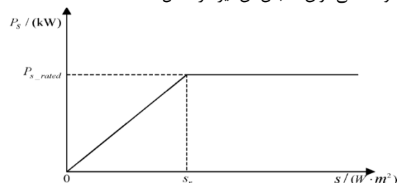
شکل (۳): رابطه بین توان خروجی و شدت تابش [۱۴]
