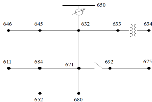
شکل (۵): شبکه استاندارد ۱۳ باس IEEE [۱۲]
