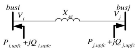
شکل (۴): مدل تزریق توان UPFC [۱۷].
