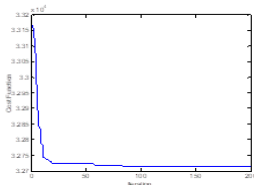
شکل (۶): نمودار همگرایی الگوریتم VCPSO برای یافتن تابع هزینه‌ی سیستم ۱۵ واحد با در نظر گرفتن مناطق عملیاتی ممنوع، محدودیت‌های رمپ ریت و تلفات شبکه انتقال
