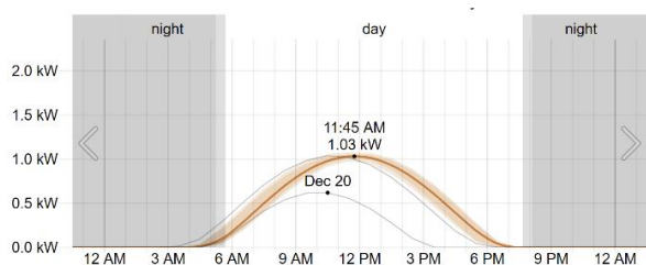
شکل (۱۳): میزان تابش خورشید در طول شبانه روز سوم
