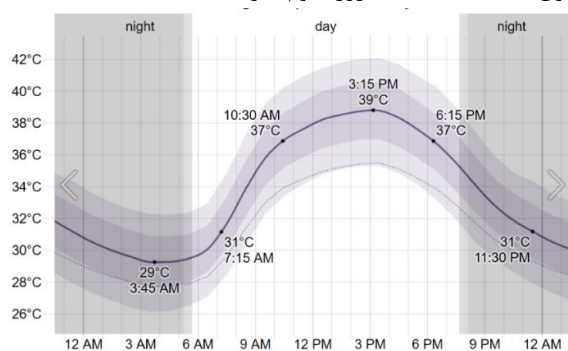
شکل (۱۲): میزان درجه حرارت شهر بم در طول ۲۴ ساعت شبانه
