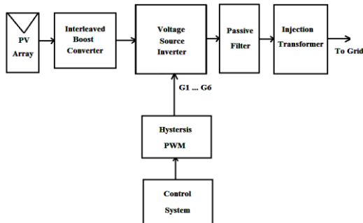
شکل (۱۱): بلوک دیاگرام کلی طرح ترکیبی بهبود یافته DVR-PV مبتنی بر چایر Interleave و مدولاسیون همسترزس
