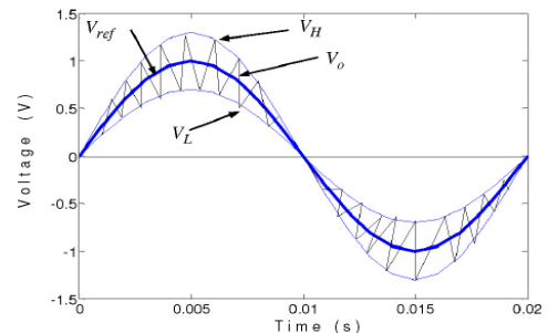
شکل (۸): اساس کار کنترل ولتاژ هیستریزس [۳۲]
