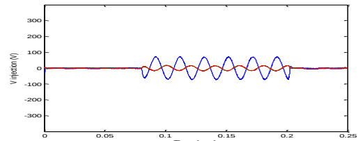
شکل (۱۴): ولتاژ تزریقی توسط جبران‌ساز در حالت وقوع کمبود ولتاژ ناشی از خطای اتصال کوتاه تک‌فاز به زمین
