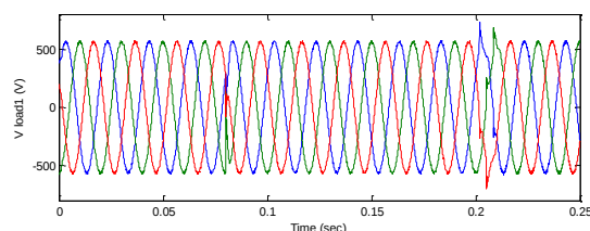
شکل (۲۲): ولتاژ سمت بار (شین ۳) در حالت وقوع کمبود ولتاژ ناشی از خطای اتصال کوتاه سه‌فاز به زمین
