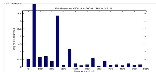
شکل (۱۷): طیف فرکانسی ولتاژ اصلاح شده سمت بار در حالت استفاده از جبران‌ساز ترکیبی مبتنی بر مبدل بوست معمولی و مدولاسیون سینوسی
