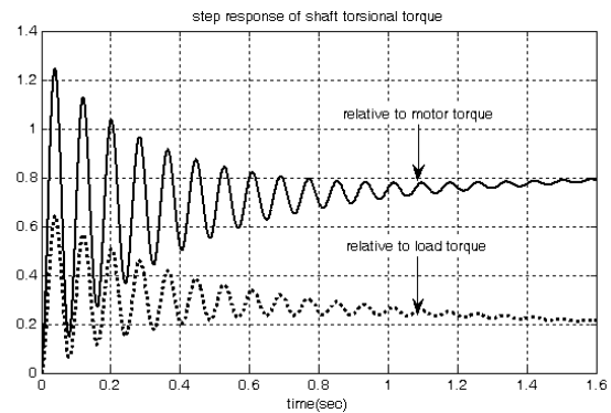
شکل (۹): پاسخ پله گشتاور پیچشی شافت به ازای تغییرات در گشتاور بار و گشتاور موتور
