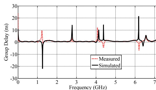
شکل (۱۱): تأخیر گروه فیلتر پوشیدنی پیشنهادی
