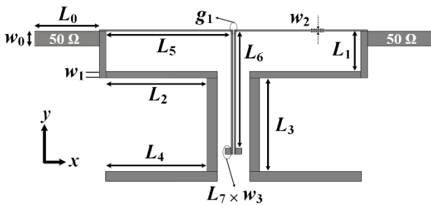
شکل (۱): هندسه‌ی فیلتر دوبانده‌ی پوشیدنی پیشنهادی
