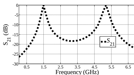
شکل ۴: پارامتر S_{21} تشدیدگرهای امپدانس پله‌ای مورد استفاده
