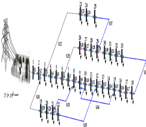
شکل (۷): شبکه ۳۳ شینه مورد مطالعه
