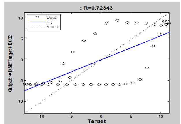
شکل ۱۴: نتایج رگرسیون برای شبکه چند لایه با لایه‌های ۳-۱۰-۲
