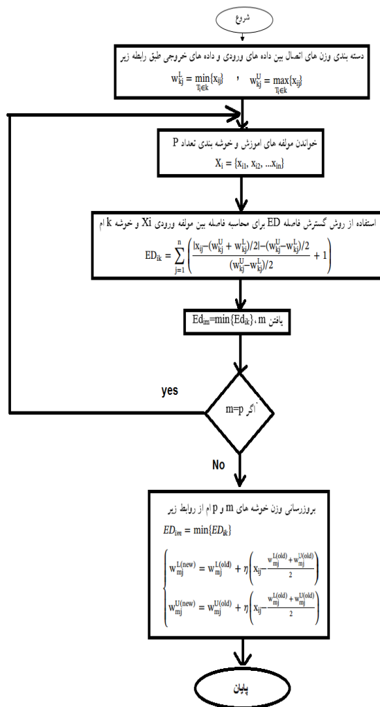
شکل ۲: فلوچارت الگوریتم شبکه عصبی تعمیمی [۲۰]
