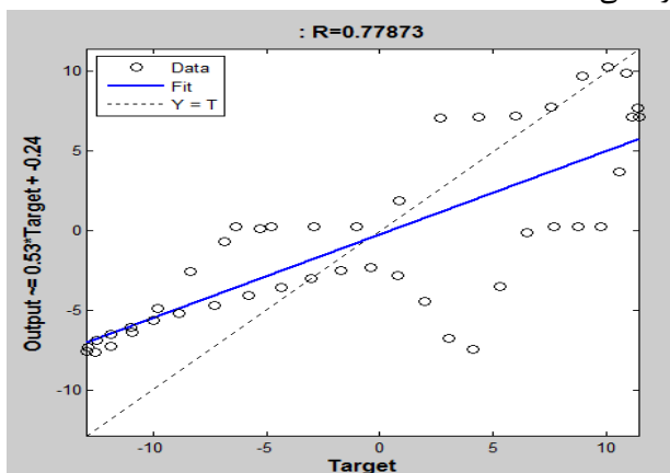
شکل ۱۳: نتایج رگرسیون برای شبکه چند لایه با لایه‌های ۲-۱۲-۳
