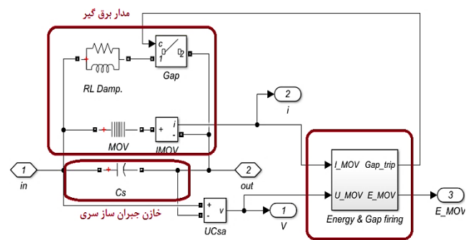
شکل (۳): شماتیک داخلی مدار خازن و حفاظت از خازن.
