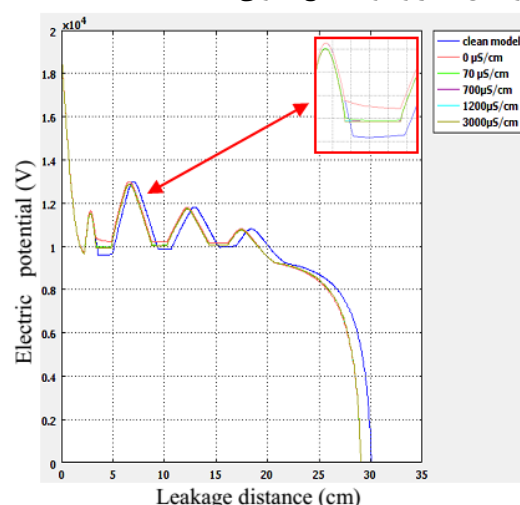
شکل (۱۸): فاصله نشت پتانسیل الکتریکی برای رسانایی های مختلف [۴۹-۵۰]
