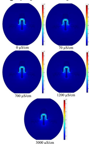
شکل (۱۹) : توزیع میدان الکتریکی برای رسانایی های مختلف [۵۴]
