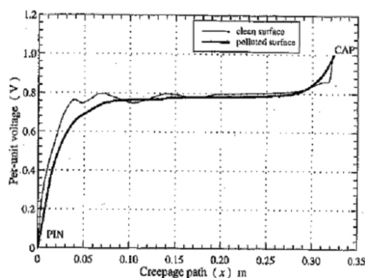
شکل (۸): توزیع ولتاژ بر روی مقره تمیز و آلوده [۳۳]
