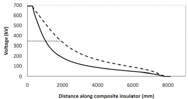
شکل (۴): توزیع ولتاژ در طول مقرر کامپوزیت برای خط 1200kV با و بدون حضور حلقه کرونا [۲۲]
