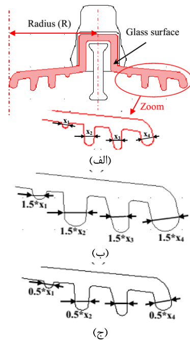
شکل (۲۲): ابعاد دنده های عایق [۵۹].
