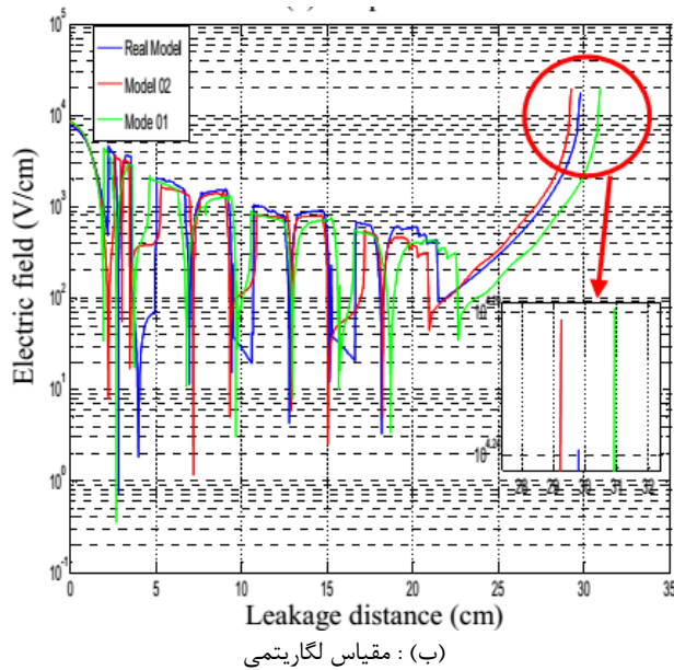
شکل (۲۳): فاصله ناشی میدان الکتریکی برای سه مورد مطالعه شده [۵۹] (مدل واقعی، مدل ۰۱، مدل ۰۲). (الف) مقیاس ساده، (ب) مقیاس لگاریتمی
