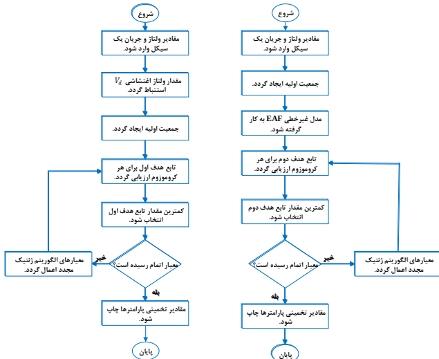
شکل (۲): اعمال الگوریتم ژنتیک بر حل مساله ی بهینه سازی
