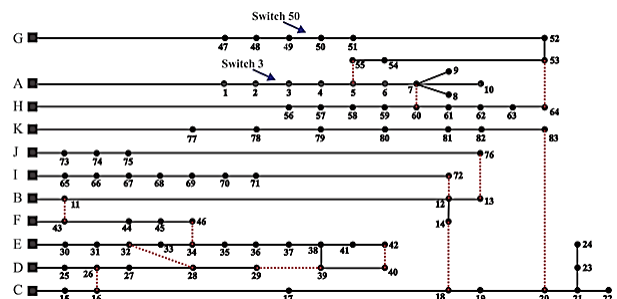
شکل (۴): دیاگرام تک‌خطی سیستم توزیع ۹۴ گره‌ای با کلیدهای مانور
