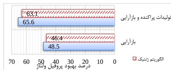
نمودار ۴-۲: درصد اصلاح پروفیل ولتاژ شین ها در بخش دوم شبیه سازی
