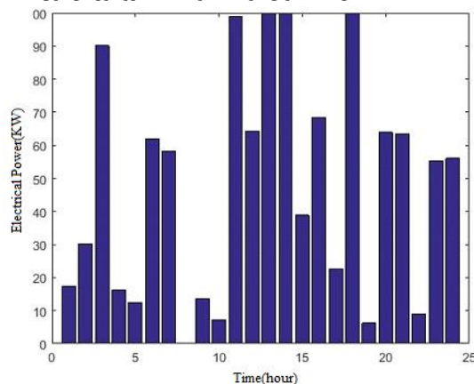
شکل (۹): توان تولیدی واحد میکرو توربین دوم
