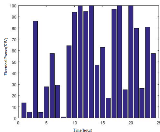
شکل (۱۰): توان تولیدی واحد میکرو توربین سوم
