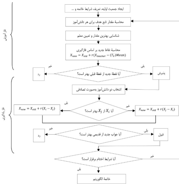
شکل (۴): فلوچارت الگوریتم TLBO [۳۷].
