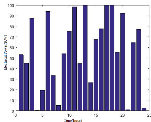
شکل (۸): توان تولیدی واحد میکرو توربین اول
