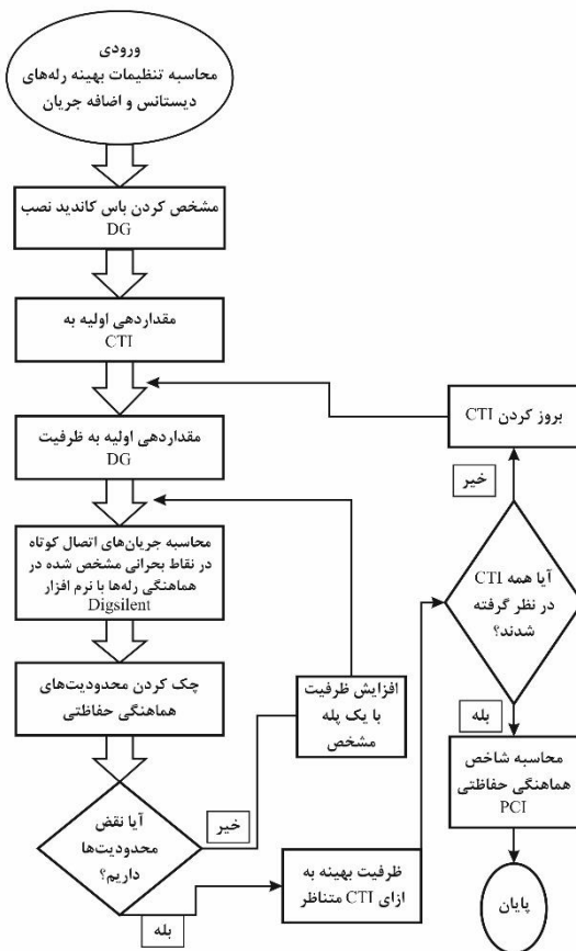
شکل (۳): فلوچارت شاخص هماهنگی حفاظتی
