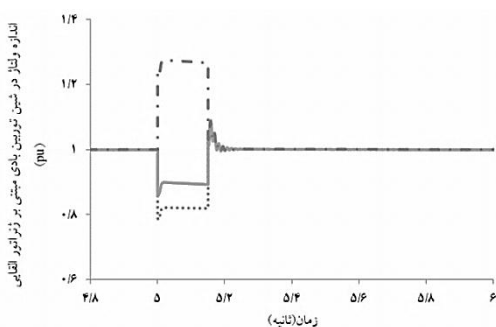
شکل (۱۲): ولتاژ لحظه‌ای rms در شین توربین بادی در اثر وقوع خطای دو فاز در ثانیه ۵ و رفع آن در ثانیه ۵/۱۵ (حالت اضافه نمودن طرح جبران کننده سری سنکرون استاتیک SSSC).
