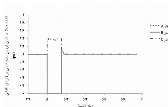
شکل (۶): ولتاژ فازهای مختلف شبکه در اثر وقوع خطای دو فاز به زمین در ثانیه ۵.
