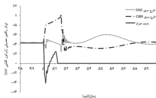
شکل (۱۹): تغییرات توان راکتیو مصرفی ژنراتور القایی خود تحریک در شرایط وقوع خطای دو فاز در حالات بدون جبران، با جبران سری SSSC و با جبران سری CSBR.
