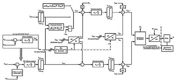
شکل (۲): مدل جبران‌کننده استاتیک سنکرون
