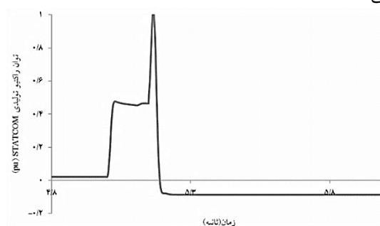
شکل (۱۰): توان راکتیو تولیدی توسط STATCOM در اثر وقوع خطای دو فاز به زمین در ثانیه ۵.
