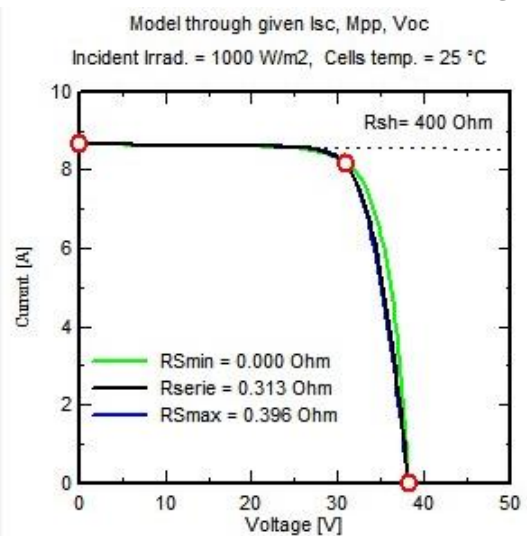
شکل (۴): نمودار I-V پنل خورشیدی
