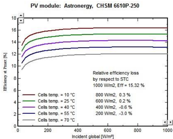
شکل (۵): دیاگرام کارایی پنل در دماهای مختلف باتوجه به تابش خورشید
