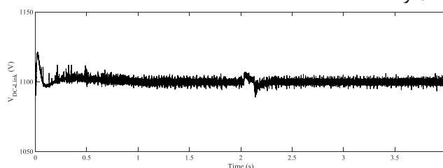
شکل (۱۱): ولتاژ لینک DC ژنراتور سنکرون مغناطیس دائم
