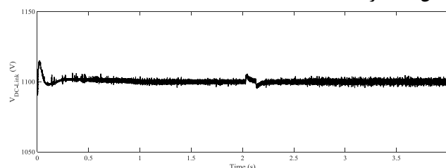
شکل (۱۲): ولتاژ لینک DC ژنراتور سنکرون مغناطیس دائم
