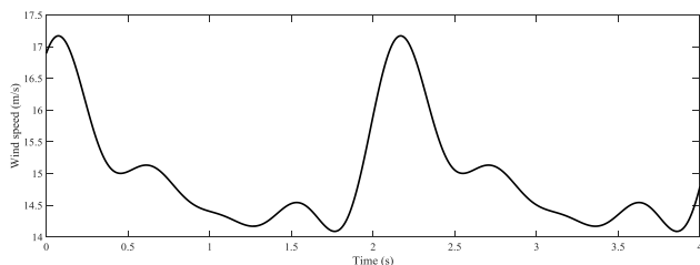
شکل (۹): تغییرات سرعت باد
