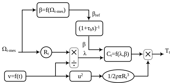
شکل (۱): بلوک دیاگرام سیستم کنترل زاویه گام
