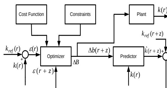
شکل (۳): بلوک دیاگرام کنترل کننده پیش‌بین مدل
