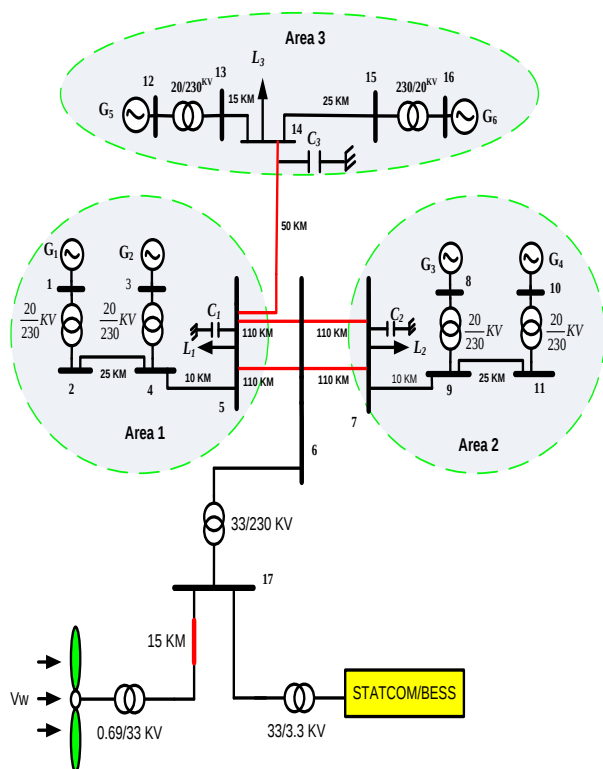
شکل (۴): بلوک دیاگرام STATCOM به همراه کنترل کننده میرایی
