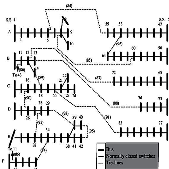
شکل (۳): دیاگرام تک خط شبکه توزیع TPC
