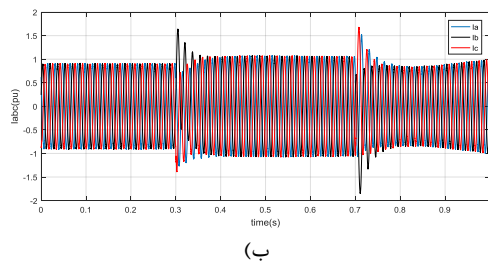
شکل (۱۲): منحنی ولتاژ و جریان بر حسب پریونیت
