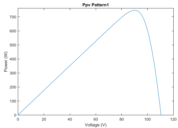
شکل (۸): نمودار توان-ولتاژ آرایه PV تحت الگوی شماره ۱
