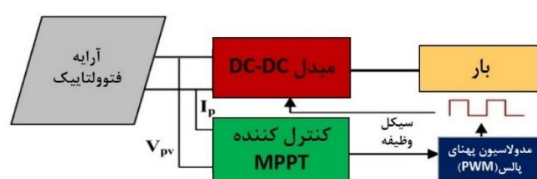
شکل (۱): بلوک‌دیگرام سیستم فتوولتائیک مستقل از شبکه همراه با
