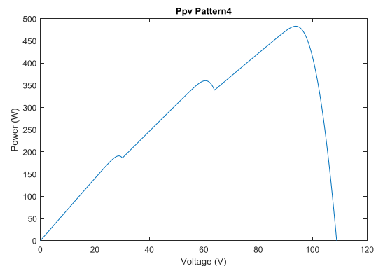
شکل (۱۴): نمودار توان-ولتاژ طبق الگوی شماره ۴
