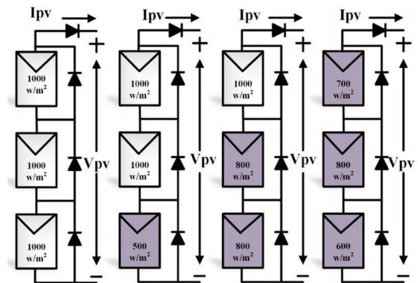
شکل (۳): پیکربندی 3s آرایه‌های خورشیدی تحت الگوهای مختلف تابش [۱۳]
