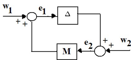
شکل (۲): مدل M - Δ
