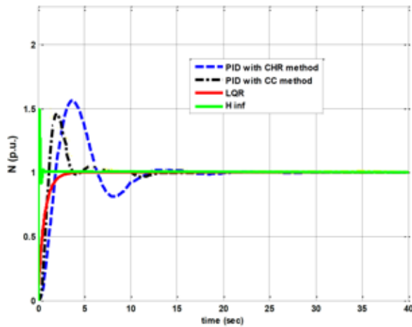
شکل ۱۱: مقایسه‌ی سرعت روتور برای CHR, CC, LQR و H_2/H_\infty
