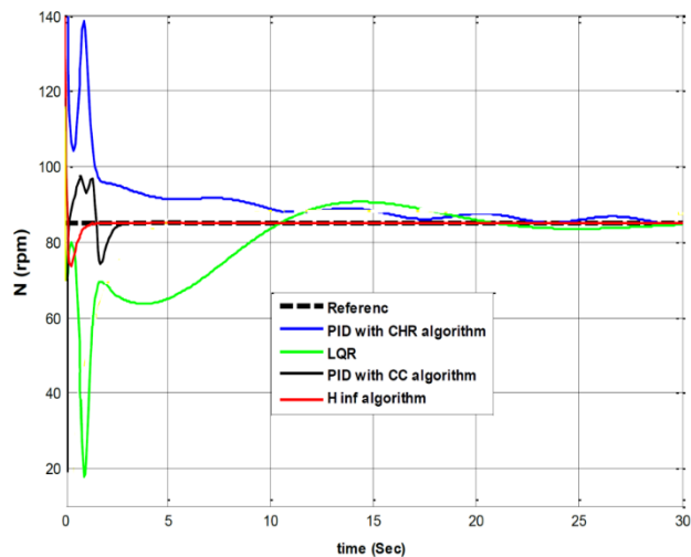
شکل ۱۳: مقایسه‌ی سرعت روتور برای CHR, CC, LQR و H_2/H_\infty با وجود اغتشاش
