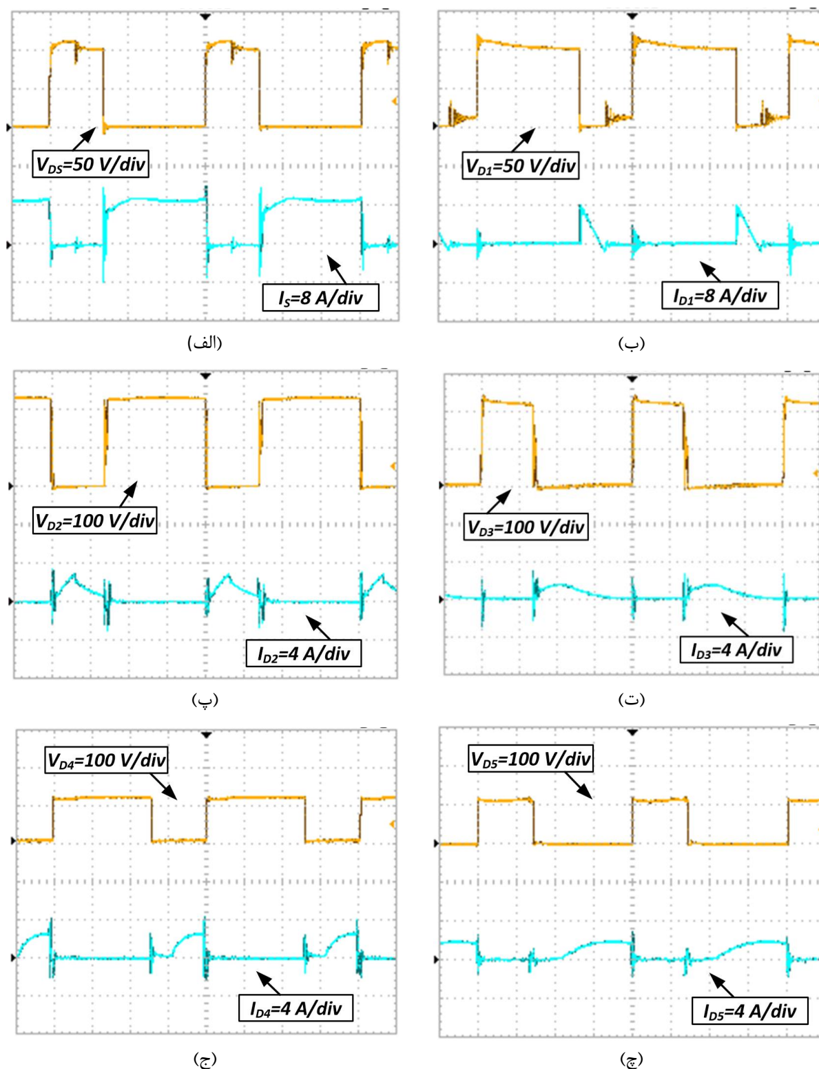
شکل (۱۲) شکل موج‌های عملی مبدل پیشنهادی
