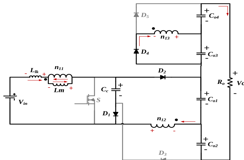
شکل (۶): مبدل پیشنهادی در وضعیت سوم عملکرد Figure (6): Equivalent circuits of the proposed converter in the third mode
