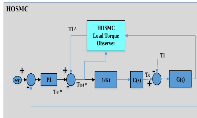
شکل ۴. بلوک دیاگرام کنترل‌کننده مبتنی بر رویت گر گشتاور بار HOSMC پیشنهادی برای حلقه سرعت IM
