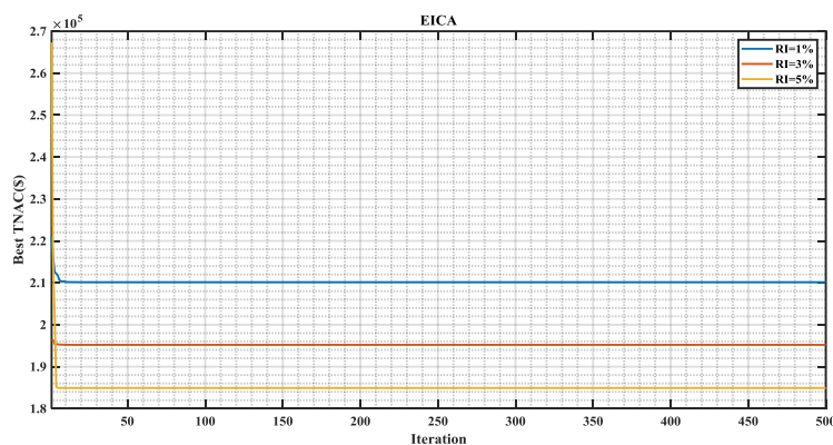
شکل (۴): منحنی همگرایی الگوریتم EICA در سه سطح RI
