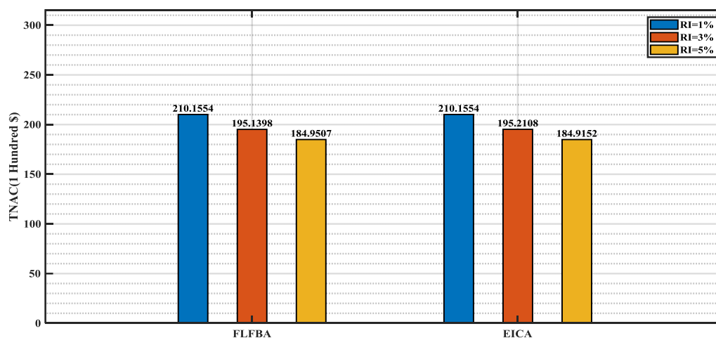
شکل (۵): مقایسه نهایی بهترین جواب هر دو الگوریتم در سه سطح RI
