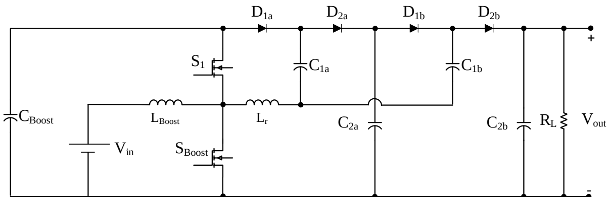
شکل (۲): نمای شماتیک مبدل رزونانسی بسیار افزاینده کلید خازنی پیشنهادی Figure (2): Schematic view of the proposed high step-up switch capacitor resonant converter.
