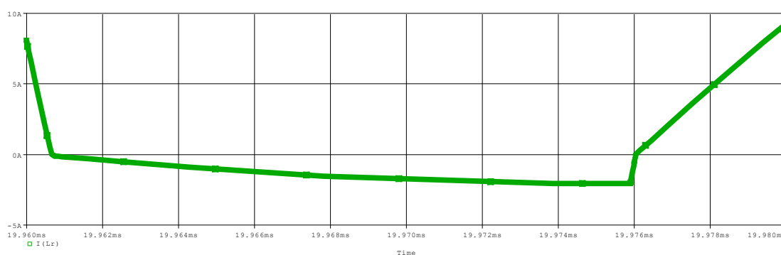
شکل (۱۰): شکل موج شبیه سازی جریان سلف L_r
