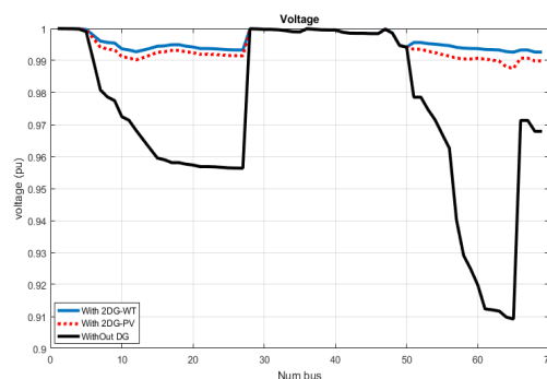
شکل (۶): تأثیر نصب دو تولید پراکنده بر ولتاژ در سیستم ۶۹ شینه
