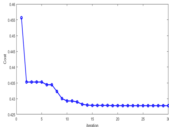
شکل (۸): منحنی همگرایی برای سیستم ۶۹ شینه با دو DG
