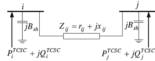
شکل (۲) مدار معادل فشرده \pi شاخه j-i با استفاده از مدل تزریق توان TCSC
