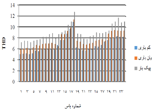
شکل (۱۲): پروفیل هارمونیکی شبکه ۳۴ شینه در حالت بدون خازن‌گذاری
