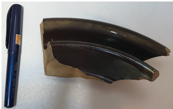
شکل (۶): نمونه‌ی مقره پس از شست‌وشو با محلول پایه
