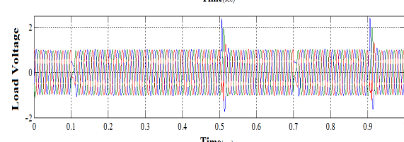
شکل (۷): شکل موج ولتاژ تزریقی توسط بازیاب دینامیکی ولتاژ و ولتاژ نهایی در فیدر بار را بعد از جبران سازی با کنترل کننده فازی بهینه
