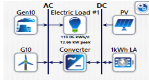
شکل (۴): بلوک دیگرام شبیه سازی شده هومر در حالت جزیره ای
