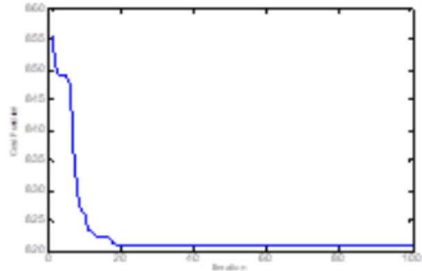
شکل (۳): نمودار همگرایی الگوریتم VCP SO برای یافتن تابع هزینهی سیستم ۶ واحد
