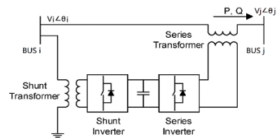
شکل (۱): نمودار شماتیک کنترل‌کننده یکپارچه توان عبوری
