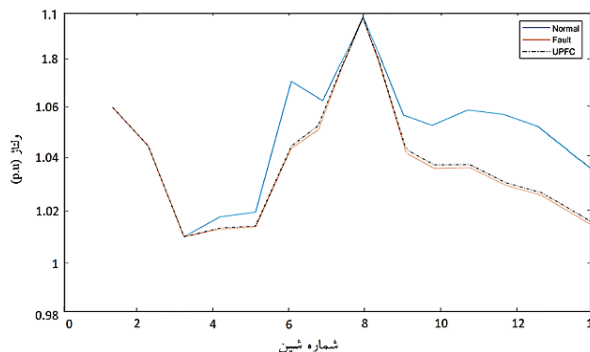
شکل (۱۱): نمودار ولتاژ در حالت خروج ژنراتور شین ۶
