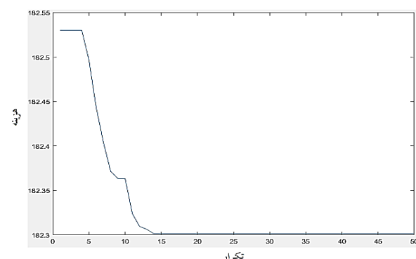
شکل (۱۶): تابع همگرایی در حالت خروج ژنراتور شین ۶
