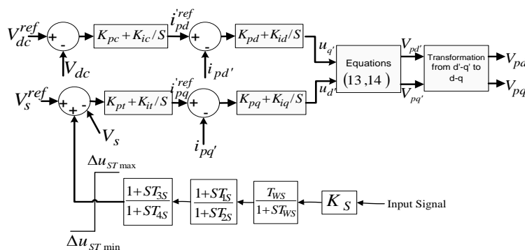
شکل (۴): ساختار کنترل‌کننده STATCOM
