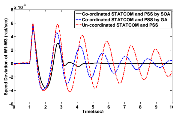
شکل (۷): تغییرات تفاوت سرعت ماشین اول و سوم برای نقطه کار اول
