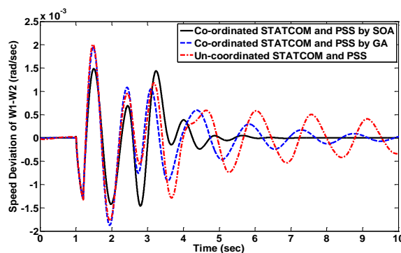
شکل (۶): تغییرات تفاوت سرعت ماشین اول و دوم برای نقطه کار اول
