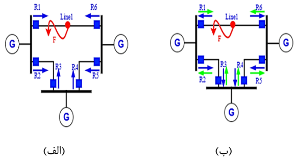
شکل (۱): الف: تمام رله‌ها از نوع DOCR متعارف است. ب: تمام رله‌ها از نوع DOCR تنظیم دوگانه است.
