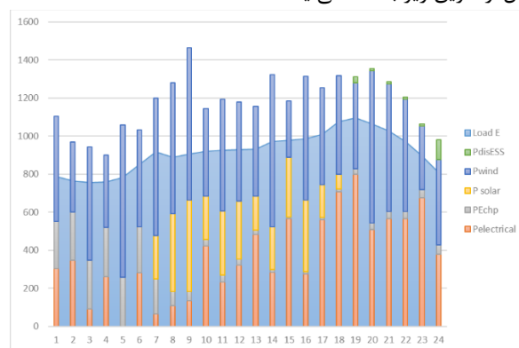
شکل ۷ پاسخ تقاضای بار الکتریکی
