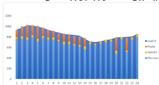
شکل ۸ پاسخ تقاضای بار حرارتی
