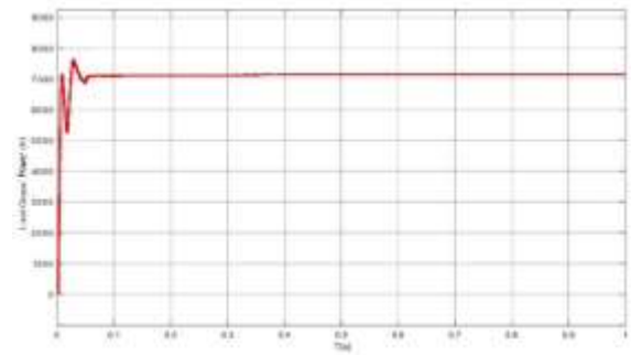
شکل ۱۷: توان بار
