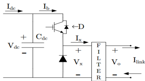
شکل (۳): توپولوژی مربوط به مبدل DC-DC
