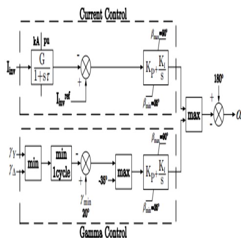
شکل (۵): ساختار کنترل‌کننده اینورترهای سیستم مورد مطالعه [۹]
