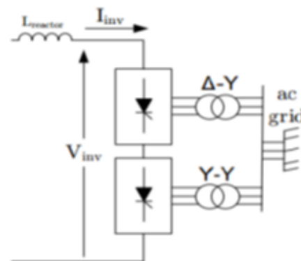
شکل (۴): نحوه اتصال نیروگاه بادی به شبکه توسط اینورتر و ترانسفورماتور
