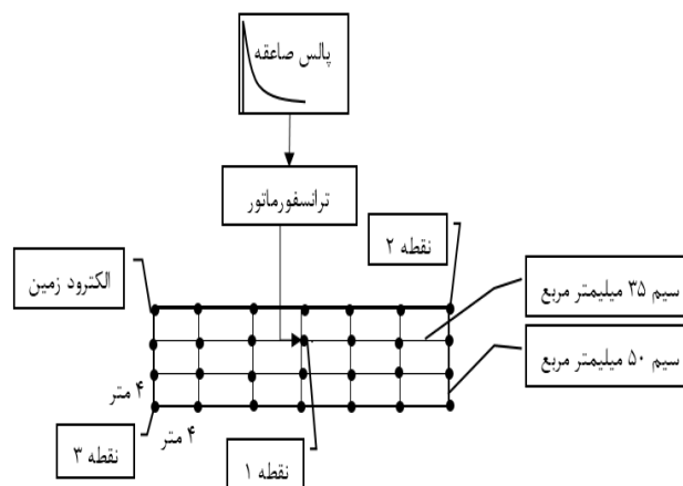
شکل (۵): جزئیات مدل خطی شبکه
