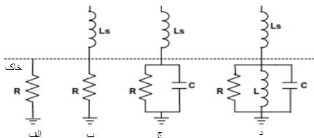
شکل (۱) مدل‌های مختلف الکتریکی میله زمین [۱۵]
